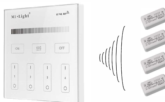
Radiofrekvenční dotykový panel pro jednobarevné led pásky. Tento ovladač je napájen AAA bateriemi a nejsou nutné žádné vodiče. Instalace na různé povrchy se zajišťuje pomocí šroubů nebo oboustrannné lepenky. Ovladač umožňuje dálkové ovládání až čtyř okruhů přijímačů nezávislých na sobě.
