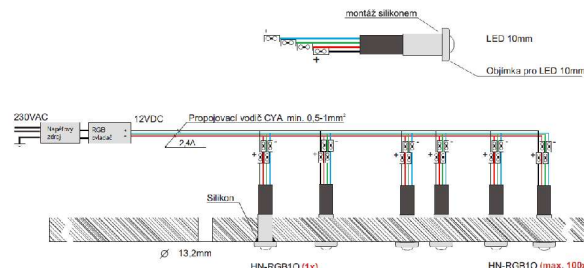
Schéma instalace - HN-RGB10 set xx ks
