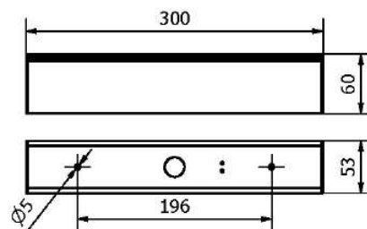
Instalace na stěnu
